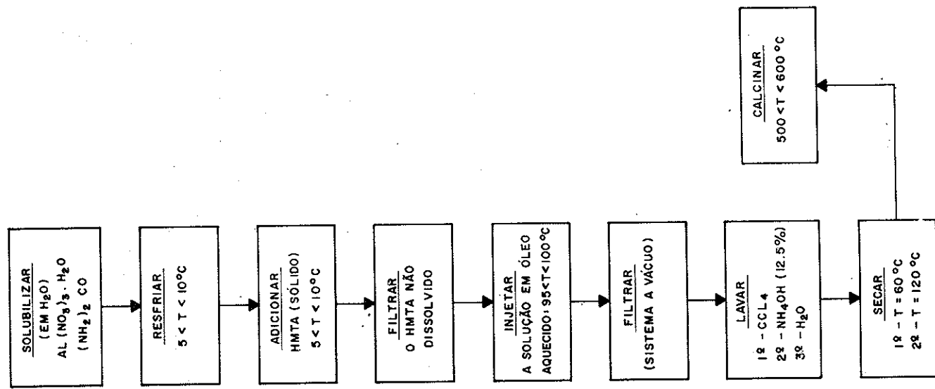
FIG. 1 — Fluxograma do processo-H (hidrólise homogênea).
