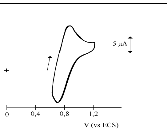
Figura 4. Voltamograma cíclico do complexo dimérico [(\text{H}_2\text{O})(\text{L})_2\text{Ru}-\text{O}-\text{Ru}(\text{L})_2(\text{OH}_2)](\text{PF}_6)_4 ( 1,00 \text{ mmol L}^{-1} ), em \text{CH}_2\text{Cl}_2 + 0,10 \text{ mol L}^{-1} \text{ Bu}_4\text{NClO}_4 , a 0,10 \text{ V s}^{-1} , eletrodo de carbono vítreo.
